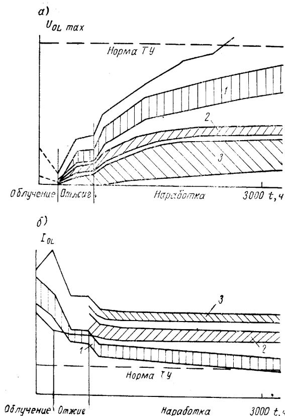
Рис. 1. Изменение параметров UOL и IOL в ходе испытаний
