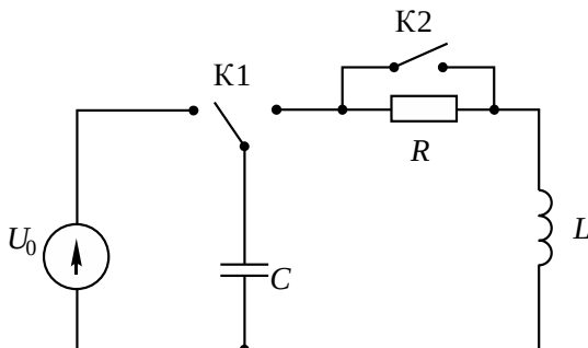
Рис. 2. Цепь вида R-C-L-O-U_0 с предварительно заряженным конденсатором до напряжения U_0 (K1 и K2 – ключ первый и второй)
