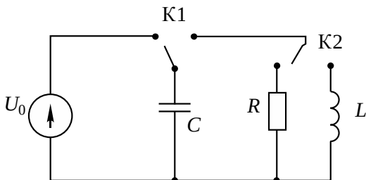
Рис. 1. Цепь вида R-C-O-U_0 с предварительно заряженным конденсатором до напряжения U_0 (K1 и K2 – ключ первый и второй)
